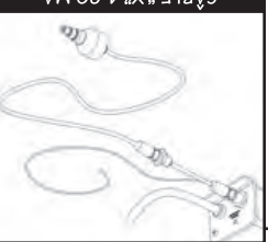
CÂBLE "Y" 4-20 MA, EN OPTION
