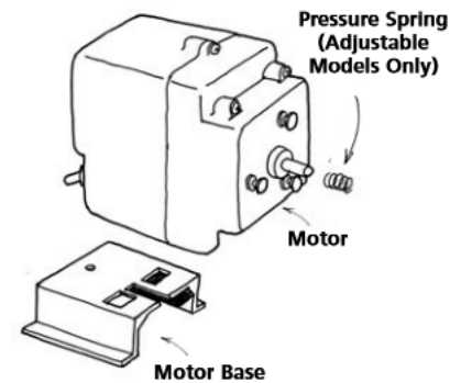
Motor Subassembly
